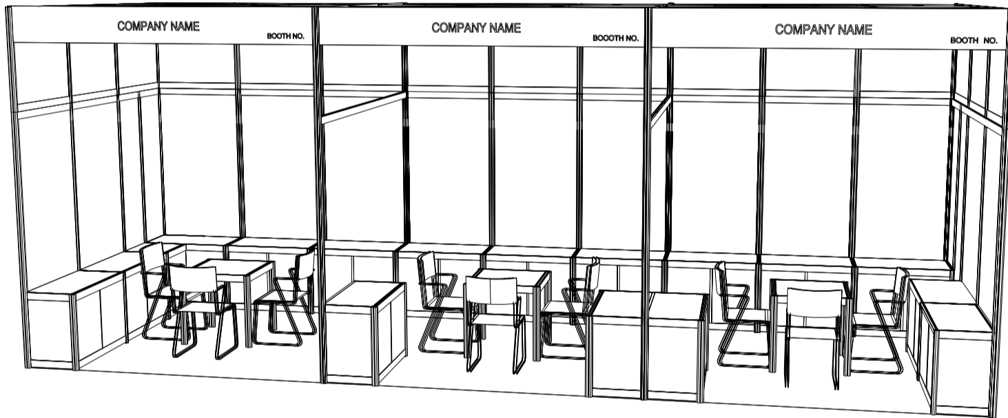
PERSPECTIVE 9M(W) X 3M(D) X 3.5M(H)
